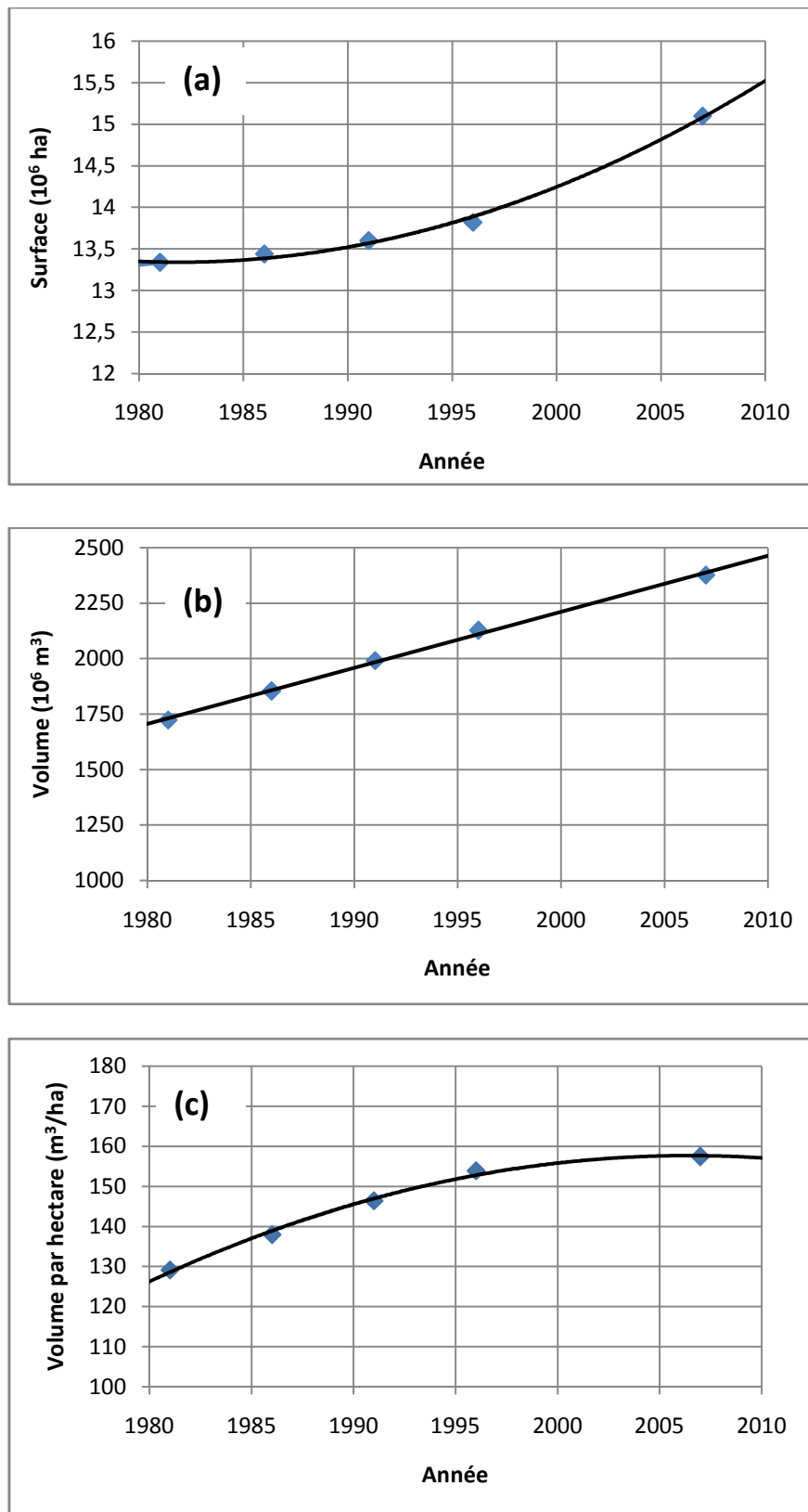
Figure 6 : Évolutions de la surface forestière de production (a), du volume total de bois sur pied (b) et du volume par hectare (c) (17)
